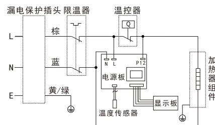
WS40\50\60\8030-K601电气原理图
