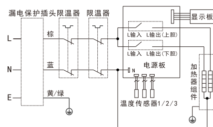
WS50\60\8033-K602电气原理图
