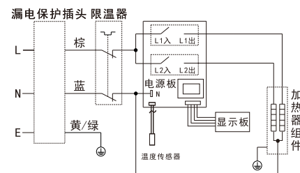
WS40\50\60\8032-K501电气原理图
