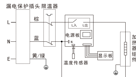
WS50\60\8032-K502电气原理图
