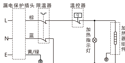
WB40(506080100)21-K202型电气原理图
