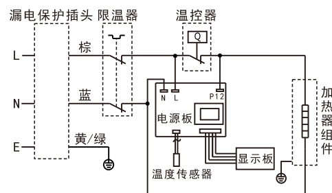
WB40(506080100)21-K202型电气原理图
