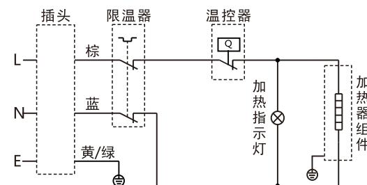
WB40(506080100)21-K203型电气原理图
